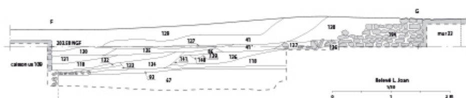
Coupe 5
