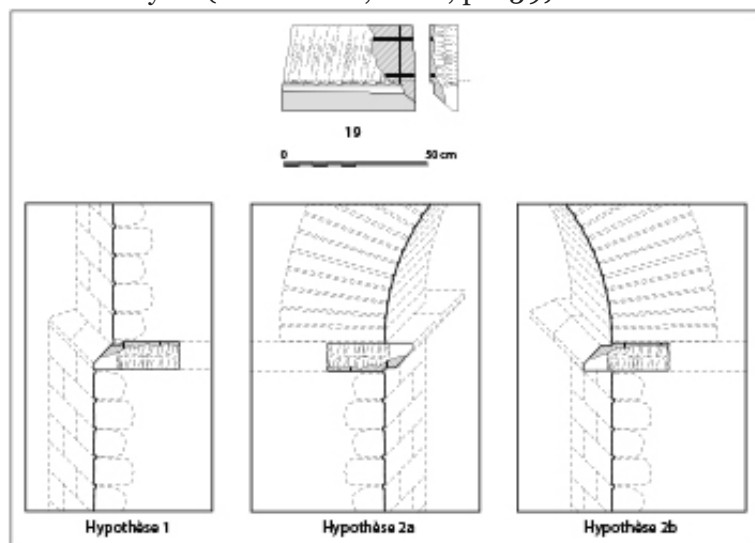
Fig. 17. Bloc chanfreiné en calcaire (n° 19) avec suggestions d'emplacement (dessin C. Gaston).
