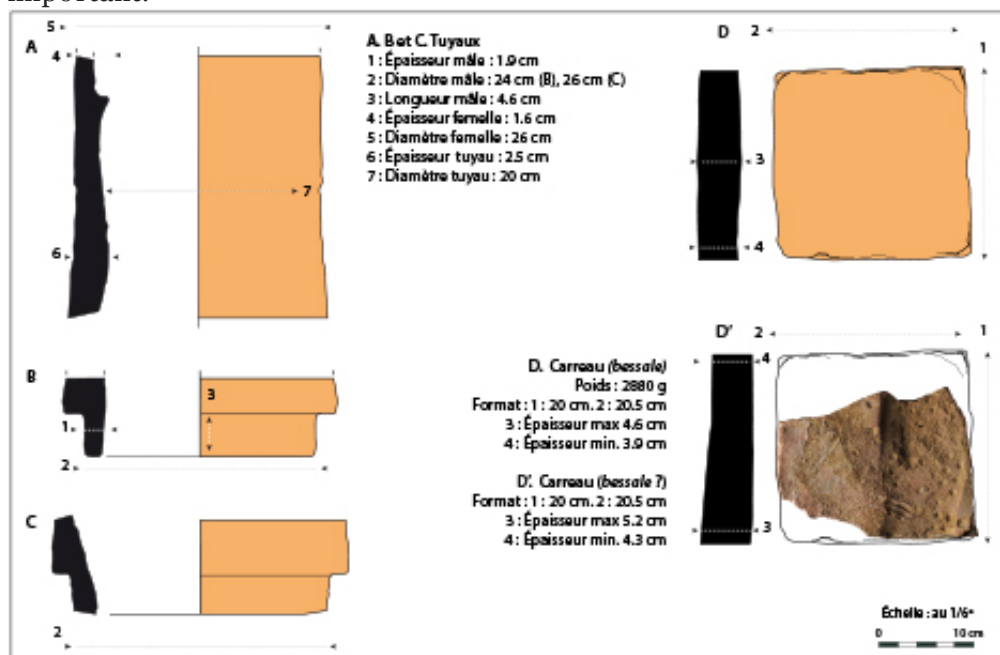
Fig. 29. Les matériaux de construction : tuyaux (A, B et C) et bessales (D) : vues de face et coupe, dimensions (photos, minutes et mises au net : S. Mouton-Venault).
