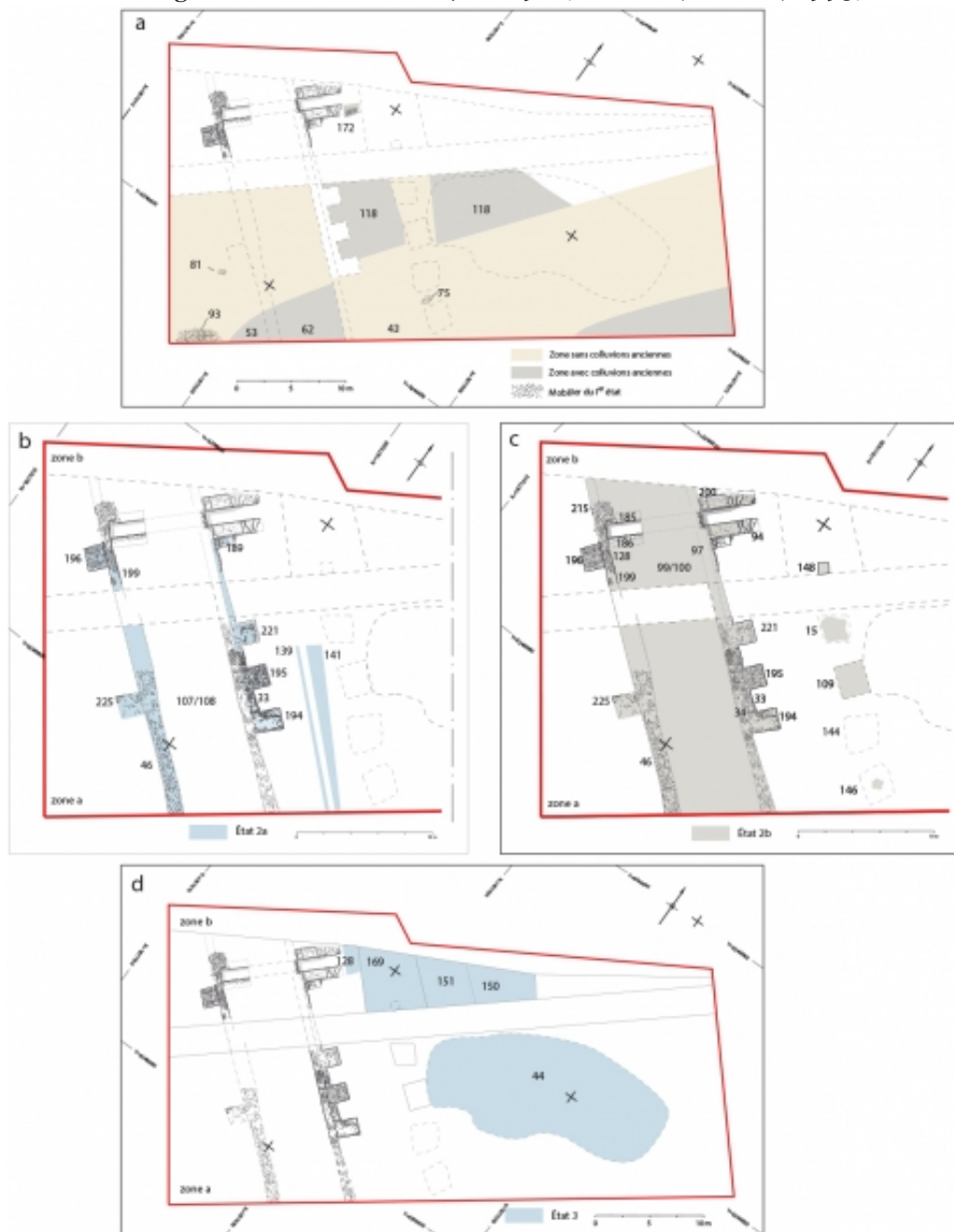
Fig. 5. Plan des états 1, 2a, 2b, 3 (D. Watts).
