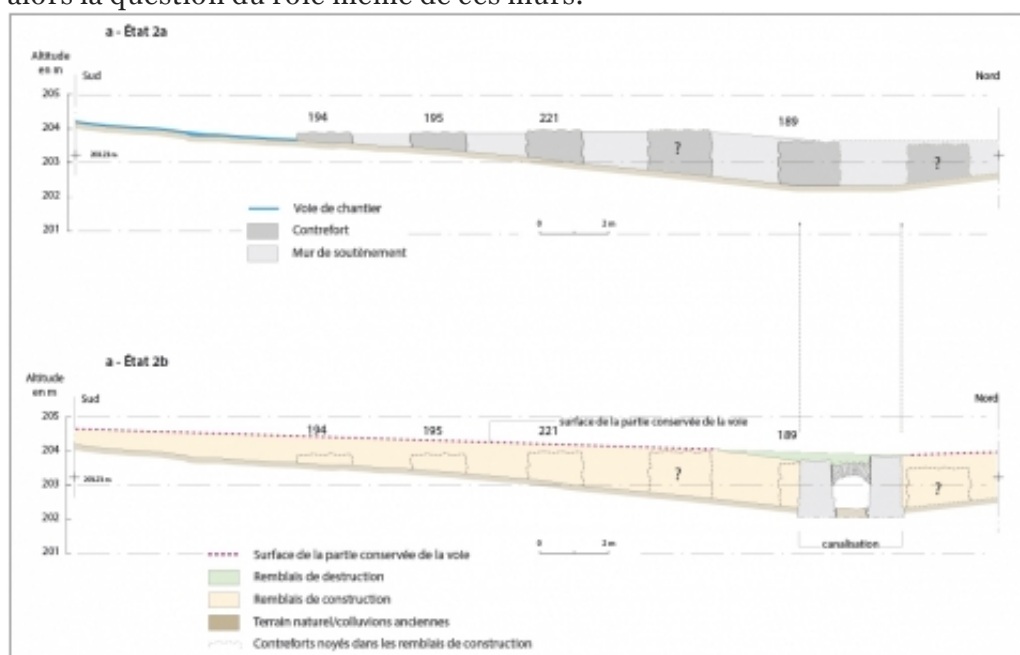
Fig. 7. Croquis de restitution de la voie dans l'état 2 (L. Joan, V. Lamy).
