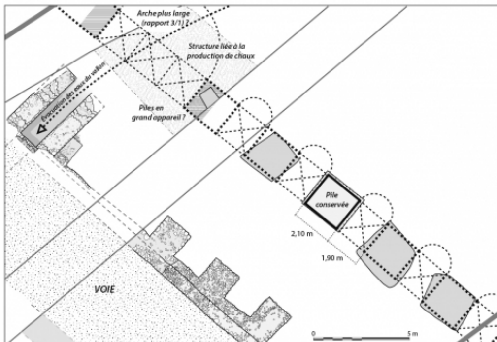
Fig. 13. Hypothèse de restitution du plan du pont-canal (dessin C. Gaston et D. Watts).
